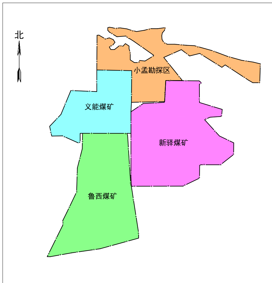
图 1-6-1 相邻矿井分布示意图
